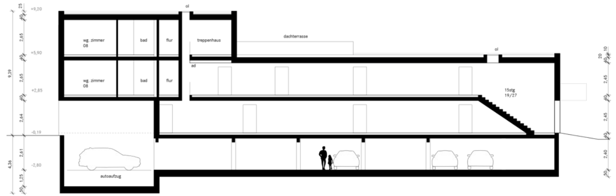
SNITT AA
