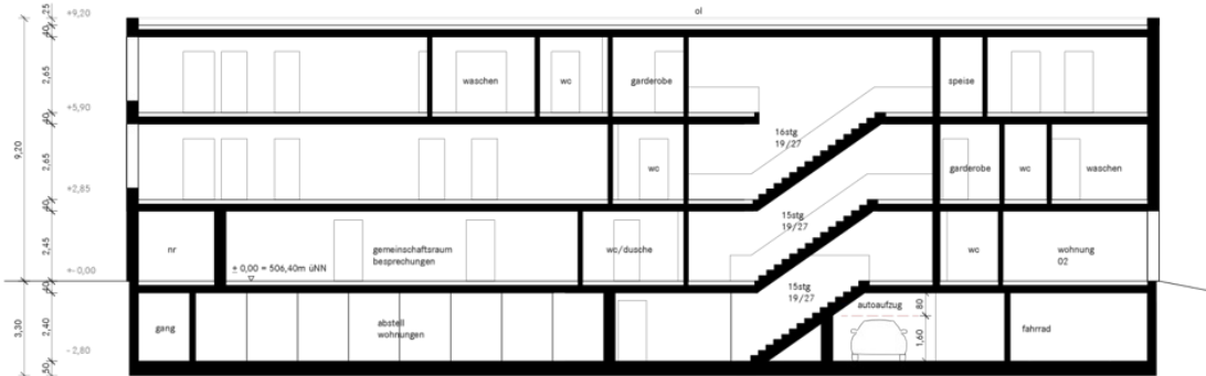
SNITT CC
